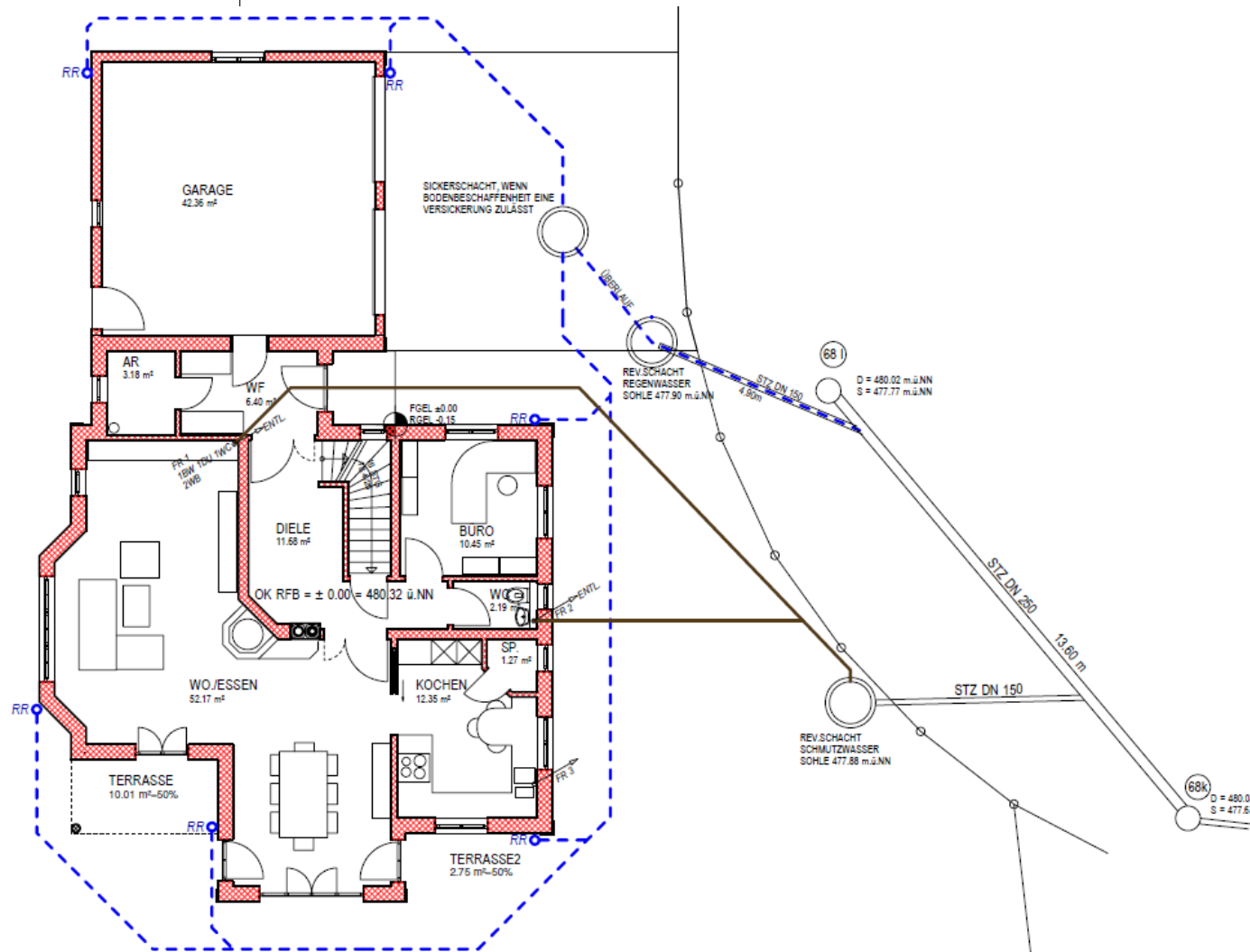
GRUNDLEITUNGEN (SCHEMA) ERDGESCHOSS
