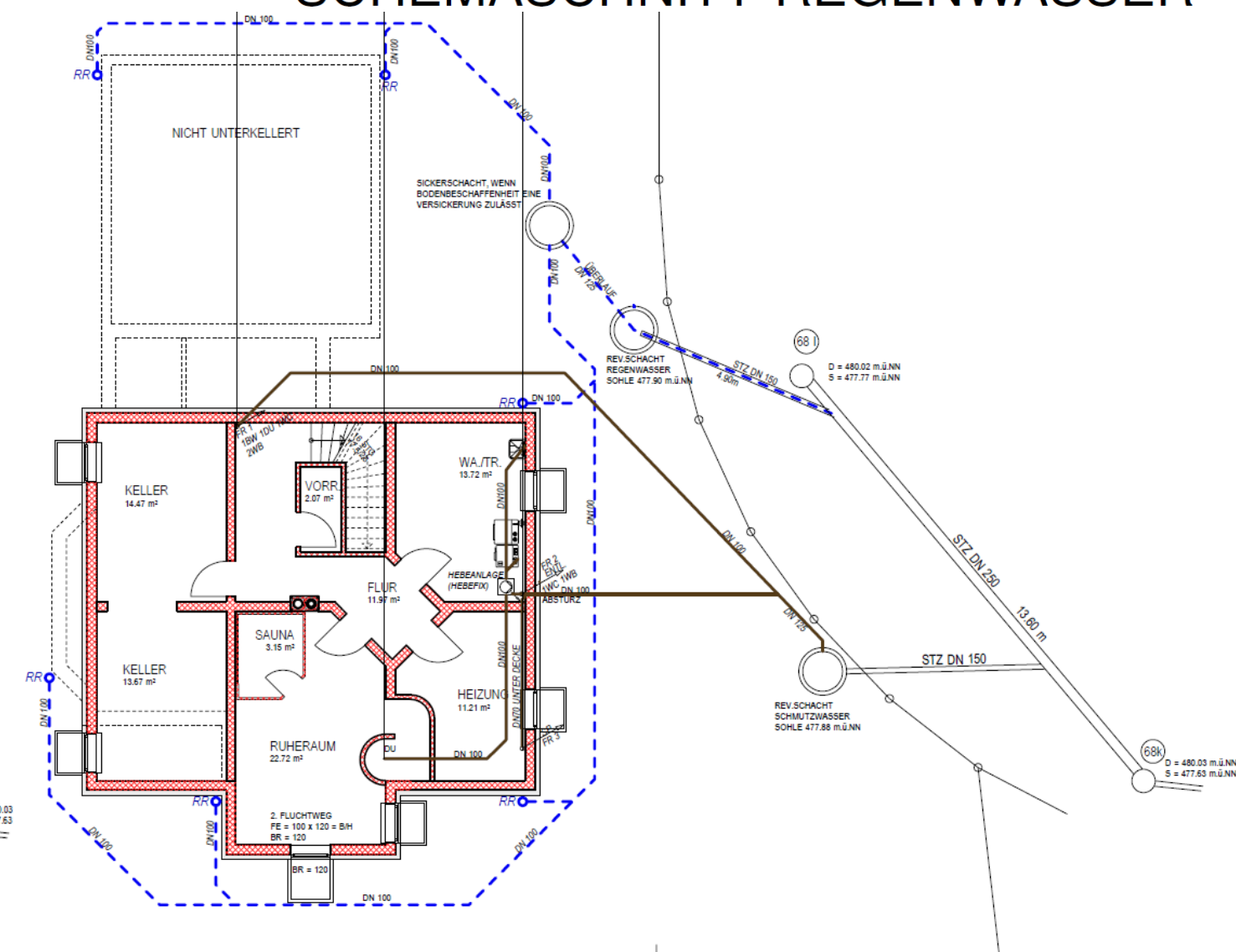
GRUNDLEITUNGEN (SCHEMA) KELLERGESCHOSS
