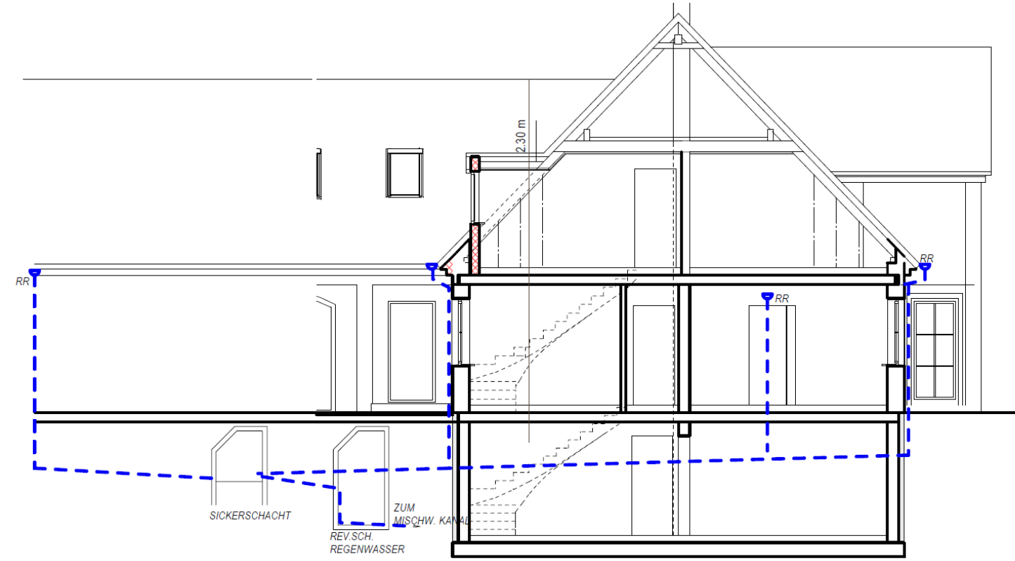
SCHEMASCHNITT REGENWASSER
