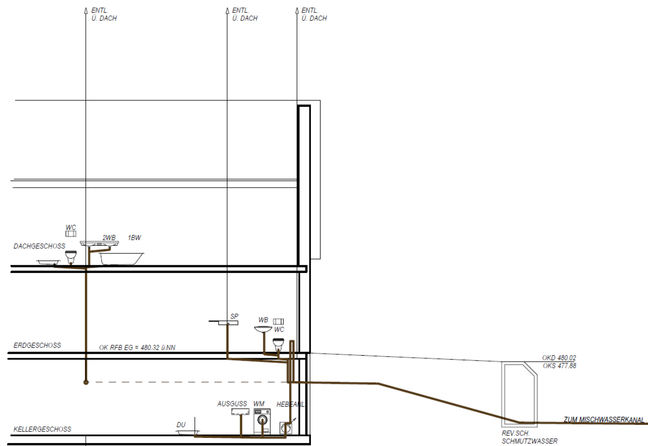
SCHEMASCHNITT SCHMUTZWASSER
